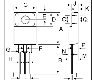
ITO-220AB
